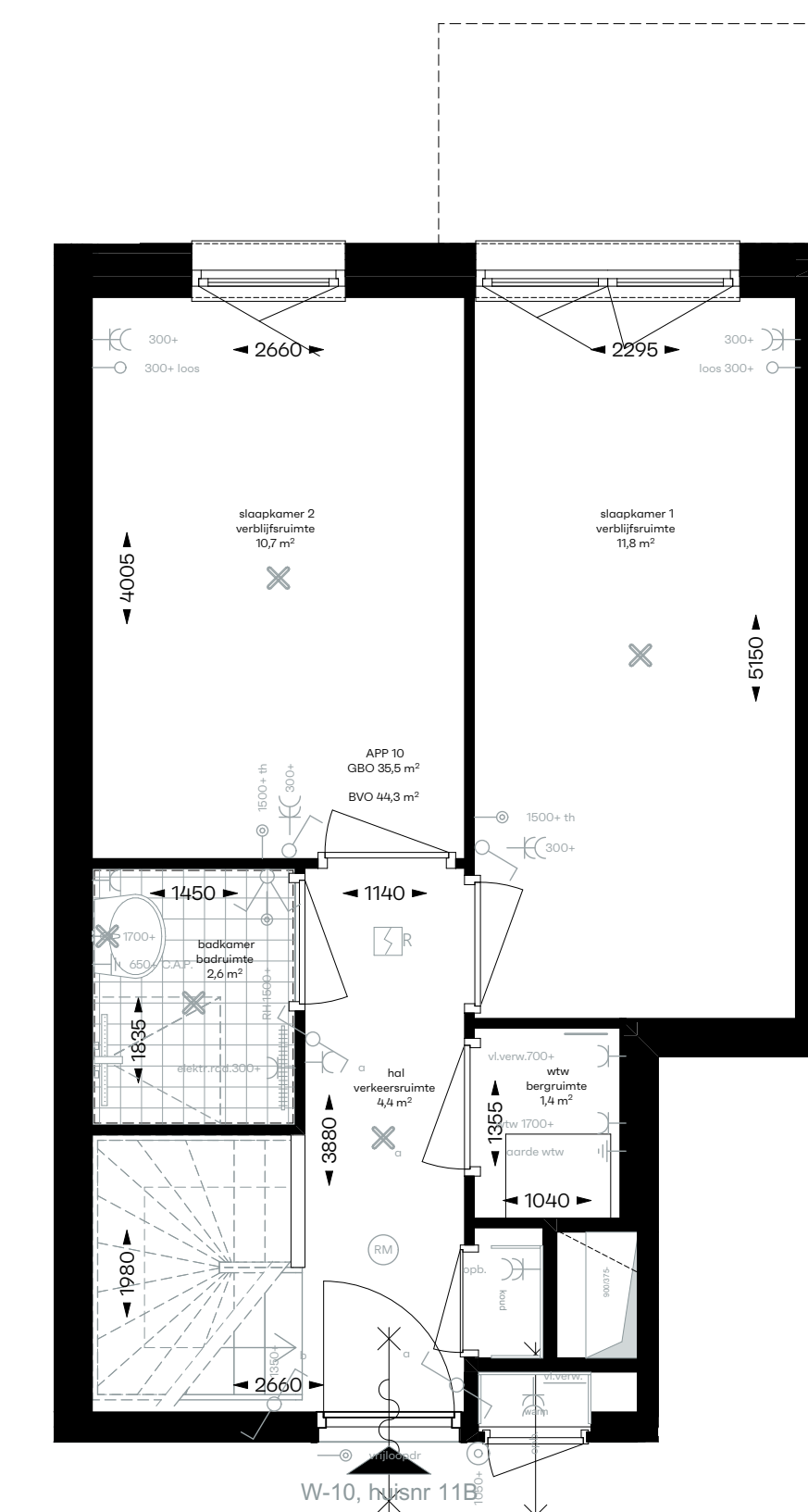
1:50 2e verdieping
