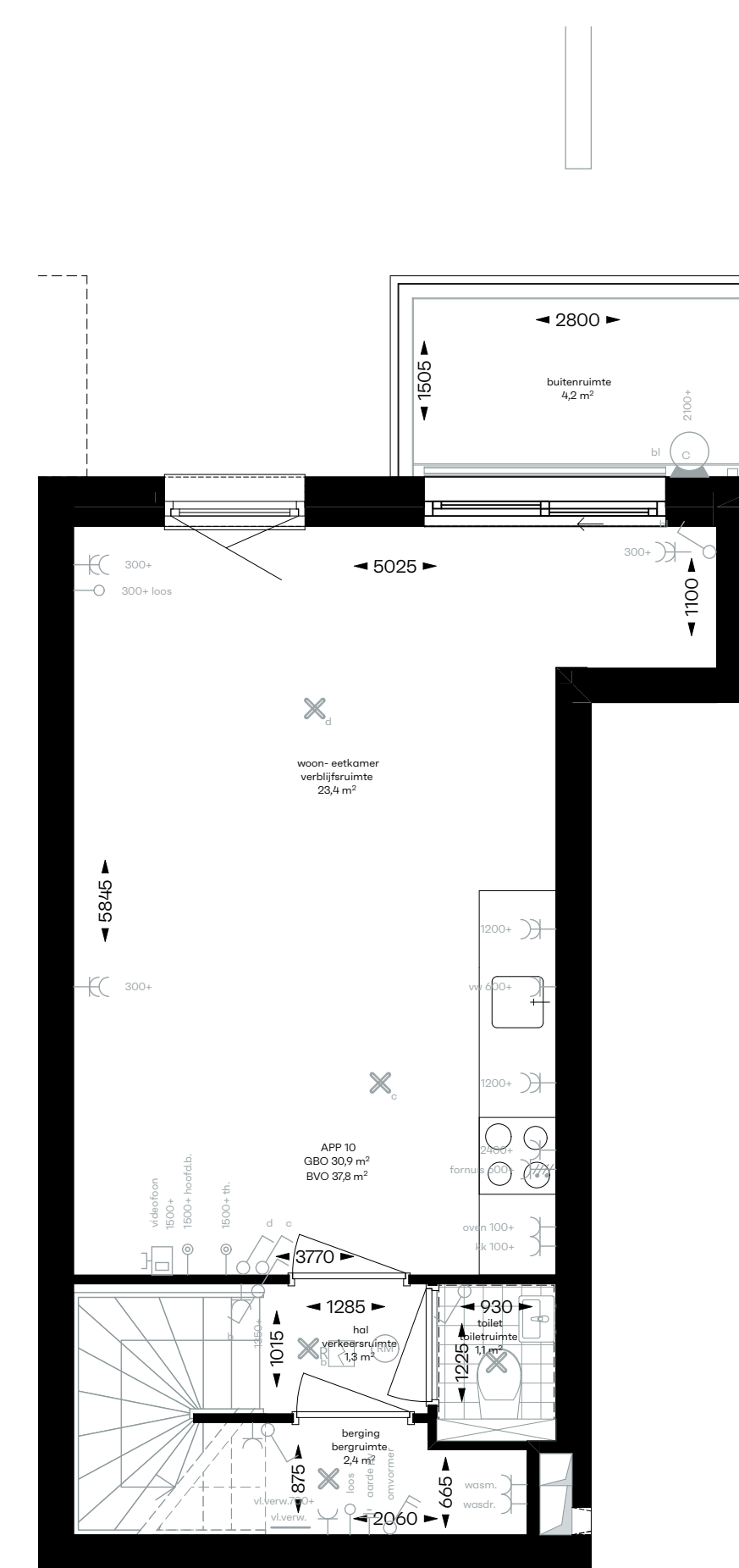
1:50 1e verdieping
